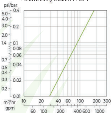
Tlakové ztráty SIGMA PRO 4"
