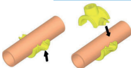
Nasadit spodní díl
