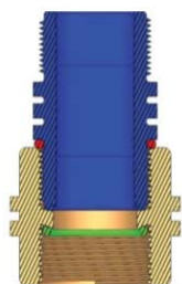
Těsnící o-kroužek u vnějšího závitu
