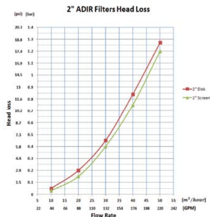
Graf tlakových ztrát pro síťový filtr 2"
