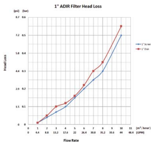
Graf tlakových ztrát pro síťový filtr 1"
