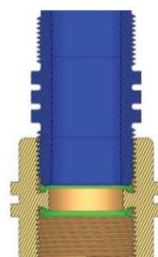
Těsnící o-kroužek u vnitřního závitu
