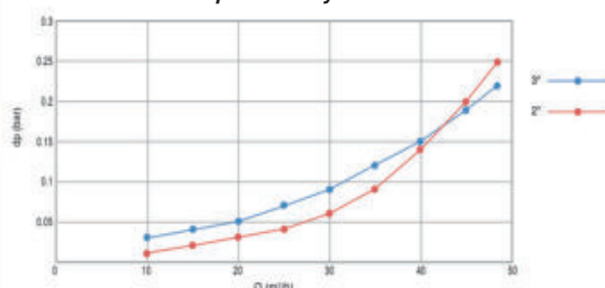
Graf tlak. ztrát pro diskový filtr 2" semi-auto
