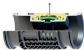
Labyrint Vstupní filtr do kapkovače
