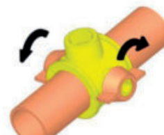
Nasadit druhou maticí a dotáhnout
